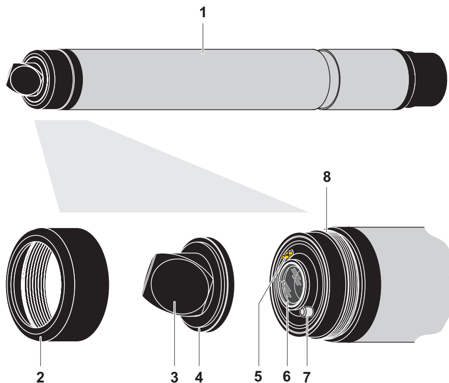
Fig. 1-1 Struttura del sensore D.O.
